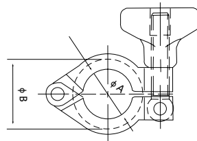
13MHH 迷你重型单销卡箍 13MHH Mini heavy duty single pin clamp SIZE: 1/2" \sim 3/4"
